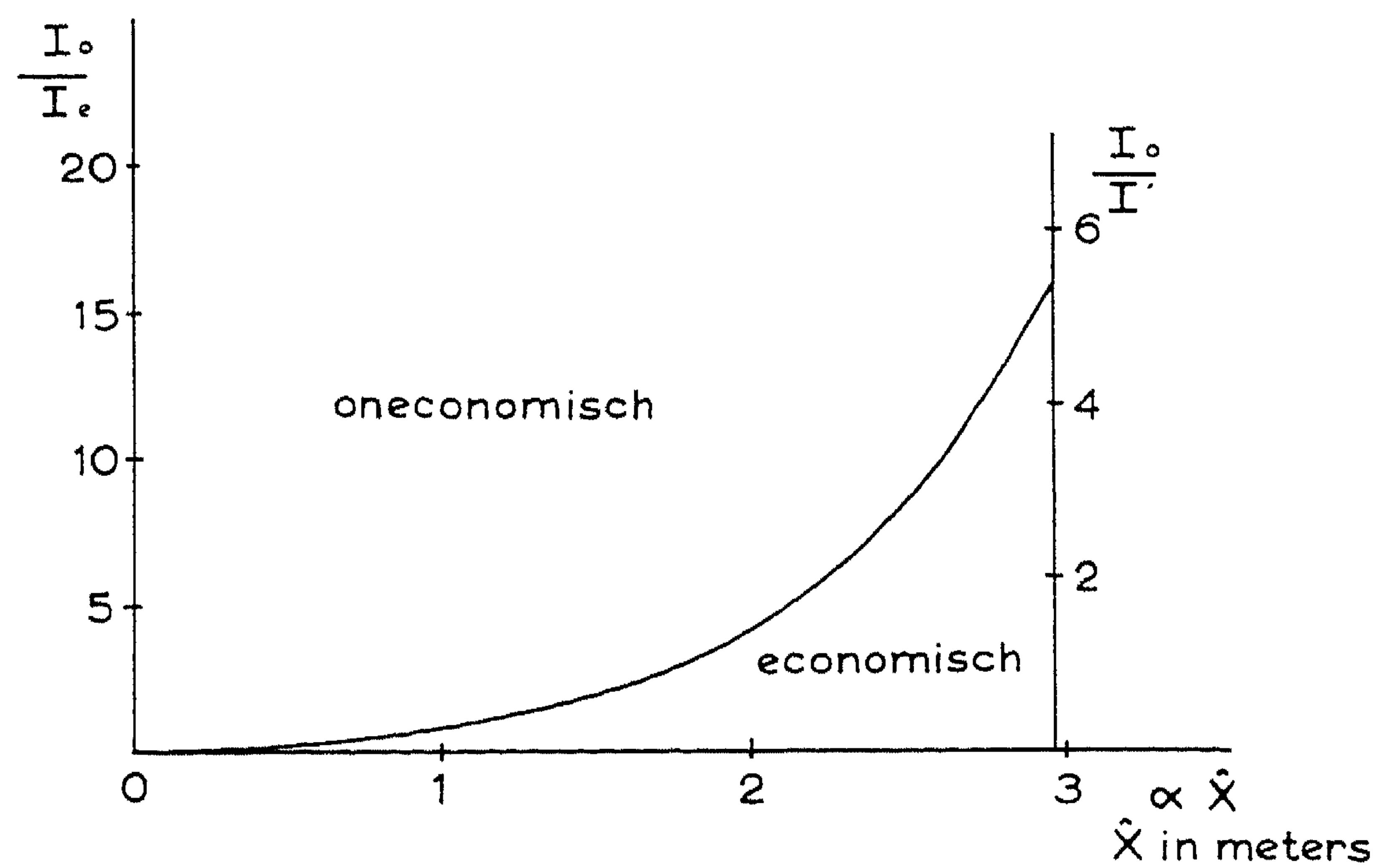
Figuur 3.2.1 Economische en oneconomische optimale dijkverhogingen
